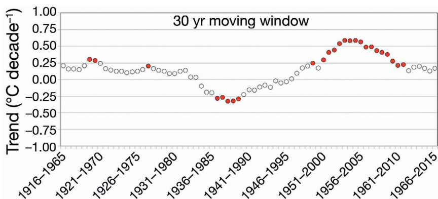
Figura 3.1. Tendencia de la tasa de valores medios anuales ( ^{\circ}\text{C/década} ) a lo largo de 30 años. Círculos rojos: p < 0,05 ; círculos vacíos: no significativo. Fuente: Sandonis et al. (2021).
