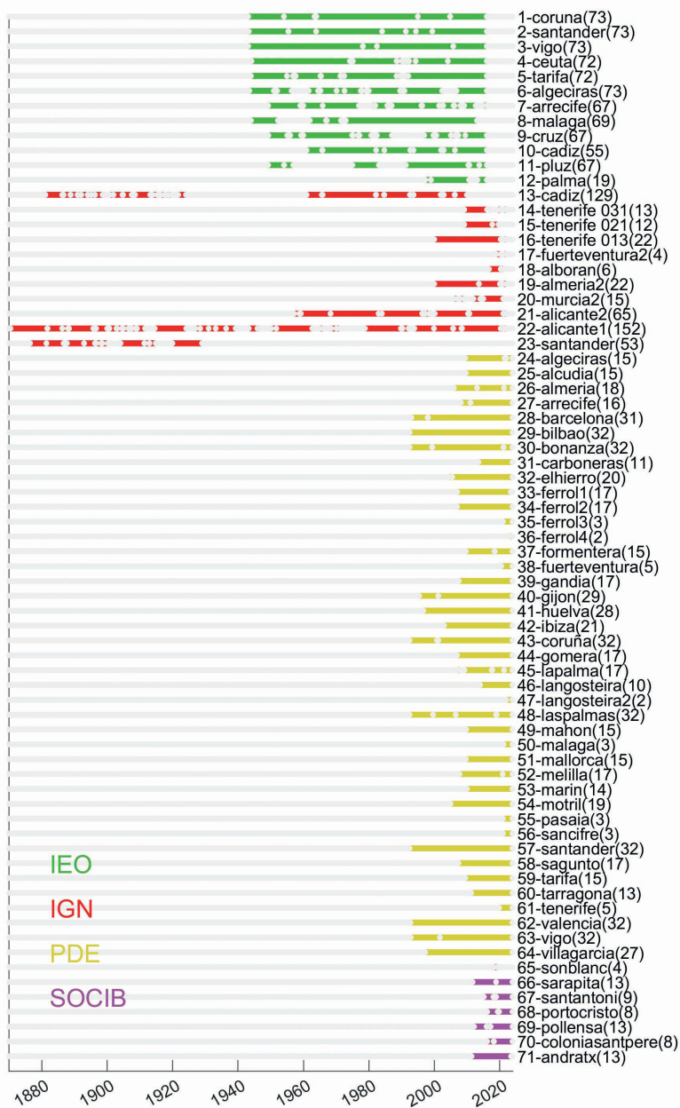
Figura 4.6. Distribución espacio-temporal de las observaciones mareográficas a lo largo de las costas españolas.
