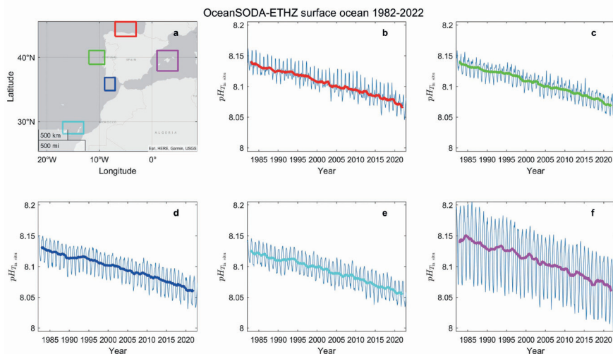
Figura 4.8. Evolución temporal del pH superficial para el periodo 1982-2022 en diferentes zonas alrededor de la Península Ibérica y Canarias. Las zonas están representadas como cuadrados en el subplot (a) y el código de color es compartido con los subplots de series temporales (b-f). Datos de OceanSODA-ETHZ (Gregor & Gruber, 2021).
