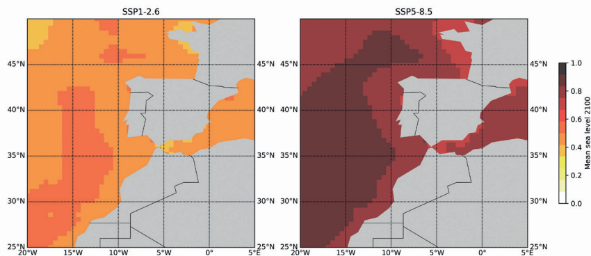
Figura 6.2. Mediana del cambio regional del nivel del mar en 2100 para diferentes escenarios (con respecto a 1995-2014) para: (Izquierda) SSP1-2.6; (Derecha) SSP5-8.5. Estos cambios incluyen todos los mecanismos que podrían evaluarse con, al menos, una confianza media (Intergovernmental Panel On Climate Change, 2023), excluyendo así los procesos de las capas de hielo asociados a una incertidumbre profunda.
