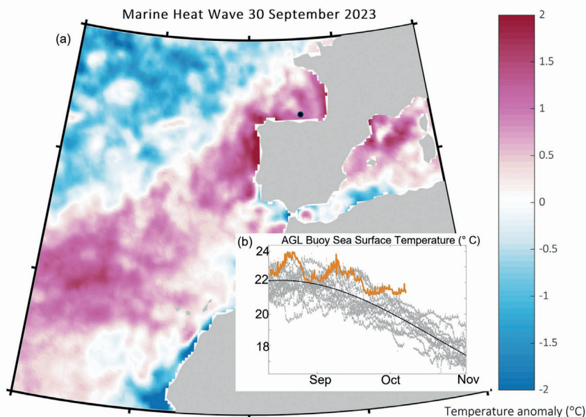
Figura 4.3. (a) Ola de calor marina en el Atlántico Norte oriental y el Mediterráneo occidental detectada a partir de datos de temperatura de la superficie del mar obtenidos por satélite (NOAA OI SST V2 High Resolution Dataset, https://psl.noaa.gov/data/gridded/data.noaa.oisst.v2.highres.html ) siguiendo a Hobday et al., 2016 a finales de septiembre de 2023, donde después del verano las temperaturas estuvieron entre 1,5 y 2°C por encima del percentil 90 de la temperatura de la superficie del mar. El punto negro en (a) marca la ubicación de la boya AGL en el Golfo de Vizcaya. (b) Temperatura de la superficie del mar registrada por la boya desde mediados de agosto hasta mediados de octubre (línea naranja) en comparación con los datos restantes registrados por la boya AGL para los mismos días del año desde su despliegue en 2007 (puntos grises) y su ciclo climatológico anual (línea negra).
