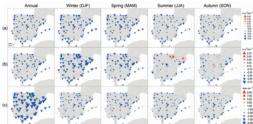
Figura 3.5. Tendencias espaciales anuales y estacionales de (a) la anomalía media mensual de la velocidad del viento cerca de la superficie (en \text{m s}^{-1}/\text{década} ), (b) la anomalía media mensual de la ráfaga de viento máxima diaria (en \text{m s}^{-1}/\text{década} ) y (c) el percentil 90 de la ráfaga de viento máxima diaria (en días/década) para 87 series de viento homogeneizadas para 1961-2019. Los triángulos rellenos azules y rojos son significativos a p < 0,05 ; los triángulos rellenos cian y magenta son significativos a p < 0,10 ; y los triángulos no rellenos no son significativos a p < 0,10 . Se han utilizado diferentes escalas para cada variable con el fin de resaltar las tendencias. Fuente: Utrabo-Carazo et al., 2022.
