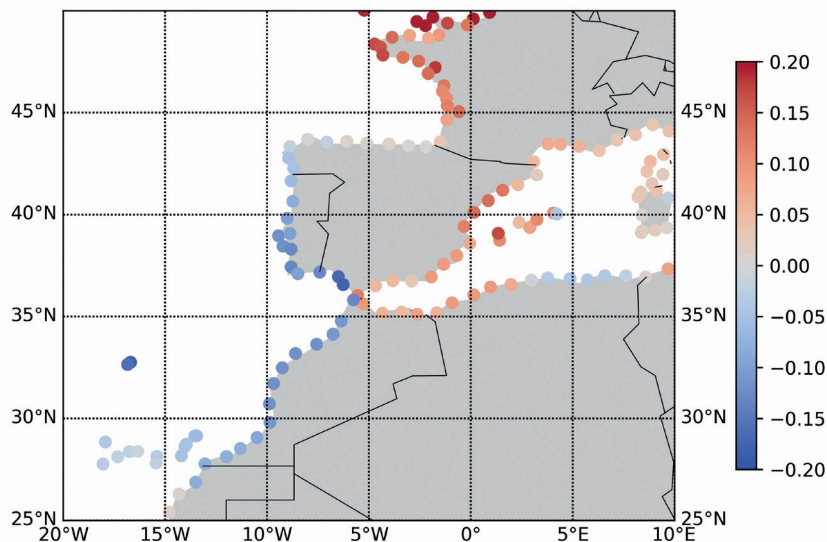
Figura 6.4. Impacto de las mareas meteorológicas y las olas en los cambios (aumento/disminución) en el percentil 95 th de los niveles extremos del nivel del mar (m) para 2100, en relación con el periodo de referencia (1980-2014) para la costa europea (adaptado de Jevrejeva et al., 2023). Esta contribución debe sumarse a la subida media del nivel del mar para obtener el cambio total de los niveles extremos.
