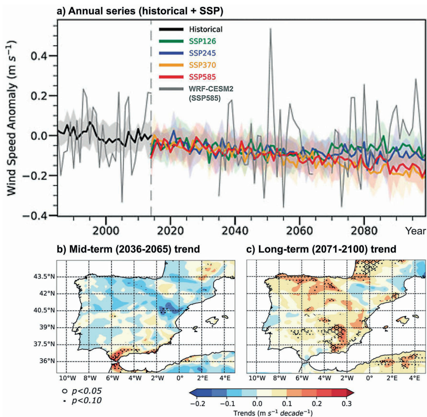
Figura 5.4: a) Anomalías anuales del NSWS ( \text{m s}^{-1} ) del MME (línea gruesa), dispersión de los modelos inter-CMIP6 (sombreado del rango entre los percentiles 25th y 75th), y el WRF-CESM2 (bajo SSP5-8.5); tendencias del NSWS ( \text{m s}^{-1} \text{ dec}^{-1} ) para b) los períodos a medio plazo (2036-2065) y c) a largo plazo (2071-2100) del WRF-CESM2 bajo SSP5-8.5. Fuente: Adaptado de Andrés-Martín y otros, 2023.
