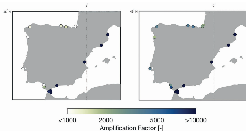
Figura 6.3. Factores de amplificación de la frecuencia media proyectada del evento centenario histórico del nivel del mar en 2100 bajo el escenario SSP2-4.5 y SSP5-8.5 (adaptado de Intergovernmental Panel On Climate Change (IPCC, 2023)). Un factor de amplificación de 100 significa que los fenómenos que se producen cada 100 años de media podrían producirse todos los años.
