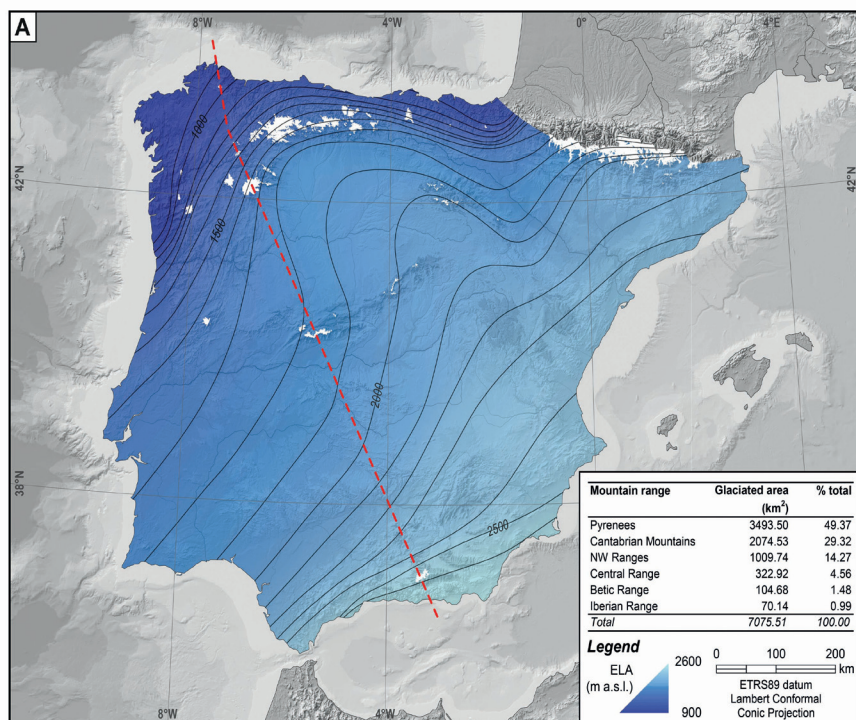
Figura 2.2. Extensión máxima de hielo en las montañas ibéricas durante el último máximo glacial (modificado de Oliva et al., 2021).
