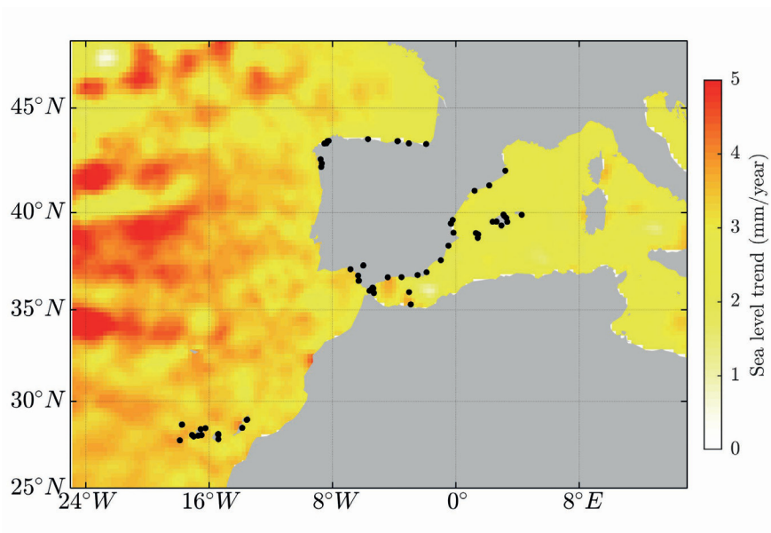
Figura 4.4. Tendencias absolutas del nivel del mar a partir de observaciones altimétricas (1993-2023) y localización de estaciones mareográficas a lo largo de las costas españolas.
