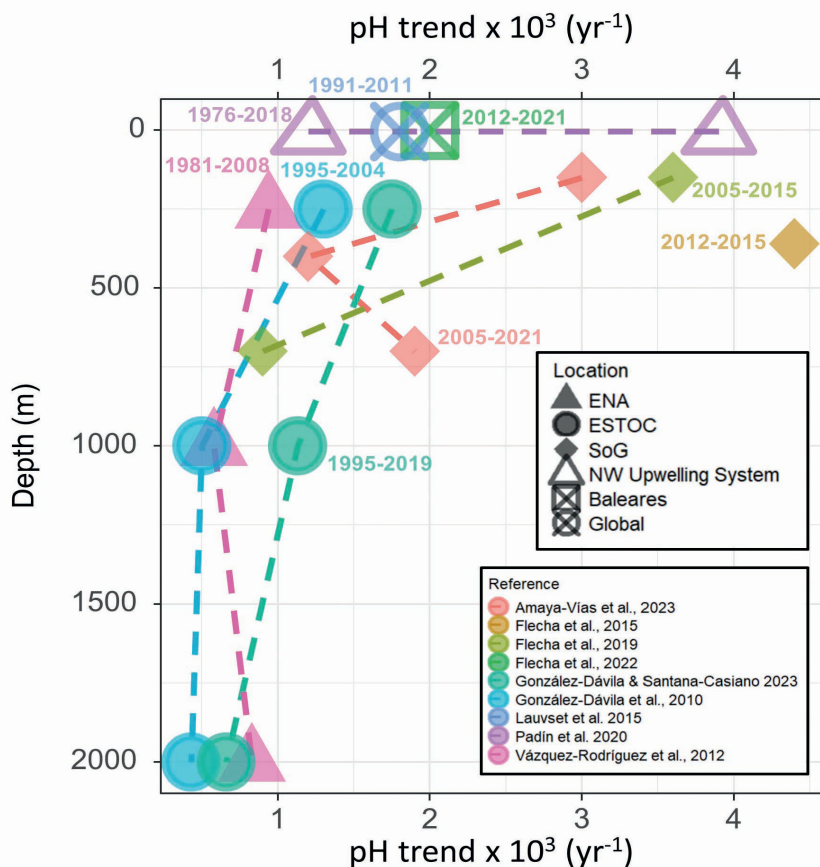
Figura 4.7. Tendencias publicadas que muestran la tasa anual de cambio del pH (unidades de pH x 10³ año⁻¹) en relación con la profundidad (desde la superficie hasta los 2000 m) para las aguas que rodean la Península Ibérica y las Islas Canarias. Los puntos de datos están codificados por colores según las referencias y conectados por líneas discontinuas para visualizar los patrones verticales. La forma de cada punto de datos corresponde a su localización geográfica. La etiqueta incluye el periodo temporal de las observaciones que sustentan la tendencia (en años).
