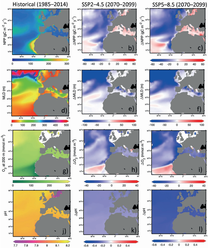
Figura 6.5. Media del conjunto CMIP6 para el periodo histórico (1985-2014) y anomalías proyectadas para el siglo XXI (2070-2099 en relación con el promedio del conjunto 1985-2014) bajo los experimentos CMIP6 SSP4-4.5 y SSP5-8.5 para (a-c) producción primaria neta, (d-f) profundidad de la capa de mezcla, (g-i) oxígeno disuelto a 200 m de profundidad, y (j-l) pH superficial. Datos obtenidos del portal web sobre cambio climático de la NOAA ( https://psl.noaa.gov/ipcc/cmip6 ).
